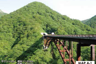
甲子大橋 (かしおおし) 甲子大橋は、一般国道289号(甲子道路)の国十交差部を架かる橋に位置する、橋長199mの長大橋です。新緑や紅葉の季節には周辺に山々を背景とした雄大な絶景が楽しめます。
